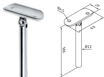
Soporte vertical para tubo redondo - regulable
