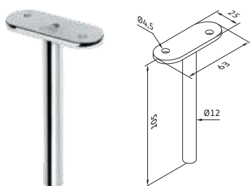
Soporte vertical para tubo plano
