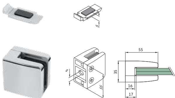
Prensacristal 55 x 55 x 35 - fijación a tubo plano con placa de seguridad
