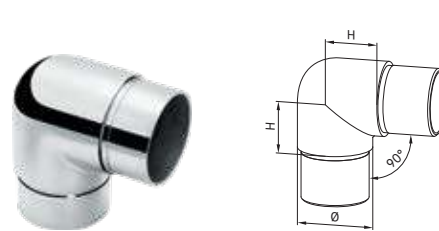
Codo conector 90° para 2 tubos
