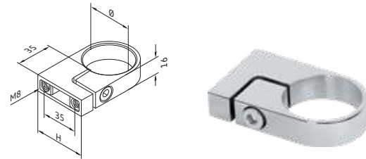
Anillo soporte para tubo redondo lateral fijación a pared
