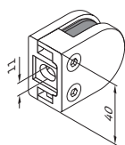
Prensacristal* 50 x 40 x 25 - fijación a tubo plano
