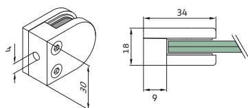
Prensacristal 34 x 30 x 18 - AISI 304 Satinado fijación a tubo plano
