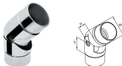
Codo conector para 2 tubos - regulable a 90° - 180°
