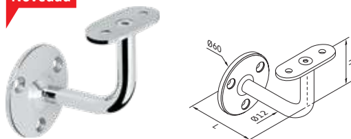
Soporte para pasamanos - tubo plano - fijación a pared
