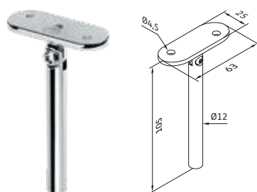
Soporte vertical para tubo plano - regulable
