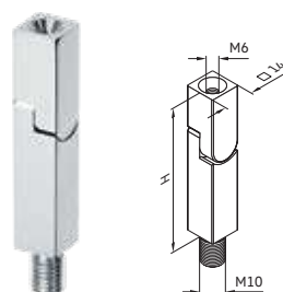
Pin cuadrado con rosca M10 - regulable
