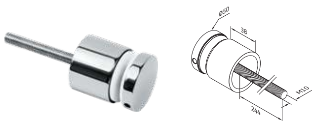
Adaptador para vidrio - fijación a pared
