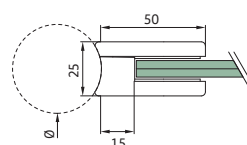
Prensacristal* 50 x 40 x 25 - fijación a tubo redondo
