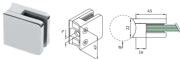
Prensacristal 45 x 45 x 22 - fijación a tubo redondo
