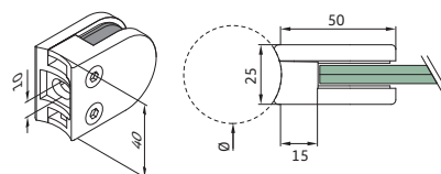
Prensacristal 50 x 40 x 25 - AISI 304 Satinado fijación a tubo redondo
