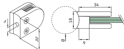
Prensacristal 34 x 30 x 18 - AISI 304 Satinado fijación a tubo redondo
