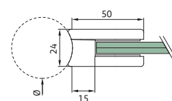
Prensacristal 50 x 40 x 24 - fijación a tubo redondo
