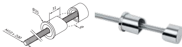
Soporte para tubo lateral - fijación a pared
