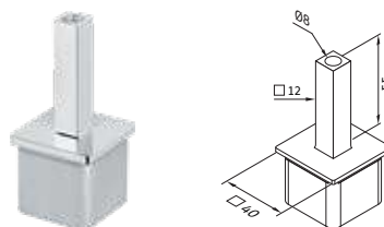
Soporte para pasamanos con rosca M8
