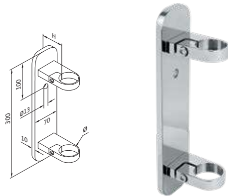
Anillo doble soporte para tubo redondo lateral fijación a pared
