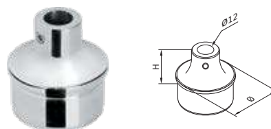
Conector a tubo para soporte vertical
