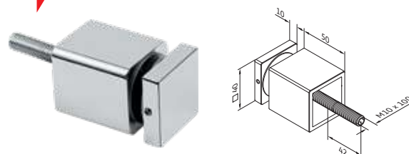
Soporte adaptador para vidrio - fijación a pared
