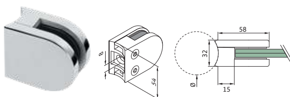
Prensacristal 58 x 54 x 32 - fijación a tubo redondo
