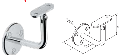
Soporte para pasamanos - tubo plano fijación a pared - regulable
