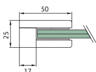
Prensacristal* 50 x 40 x 25 - fijación a tubo plano
