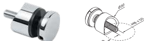
Adaptador para vidrio - fijación a tubo redondo
