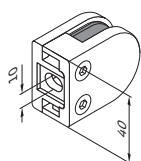
Prensacristal 50 x 40 x 24 - fijación a tubo plano
