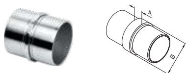
Conector para 2 tubos
