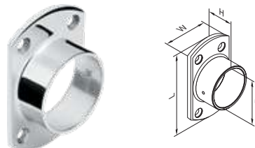
Soporte para tubo redondo - fijación a pared
