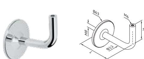
Soporte para pasamanos con rosca M6 - fijación a pared solo varilla
