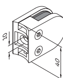
Prensacristal 50 x 40 x 24 - fijación a tubo redondo
