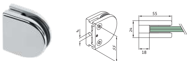
Prensacristal 55 x 18 x 24 - fijación a tubo plano
