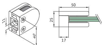
Prensacristal 50 x 40 x 25 - AISI 304 Satinado fijación a tubo plano
