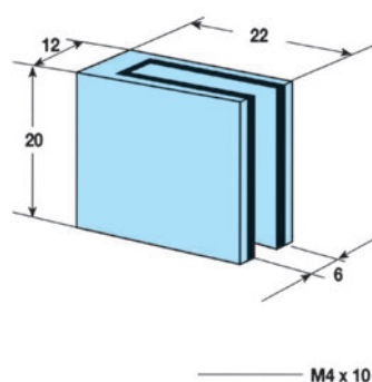
Fijación vertical FV / Vertical fixing FV
